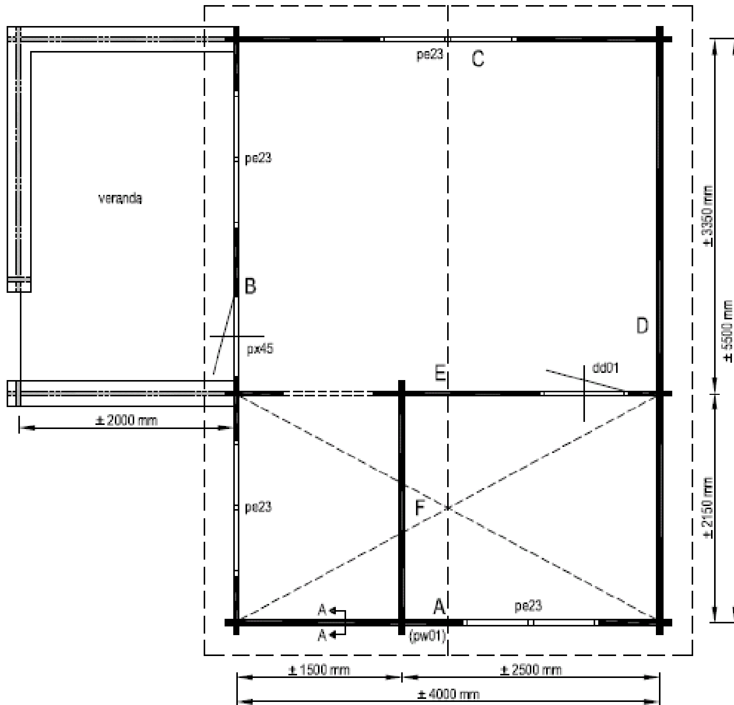
Grondplan
