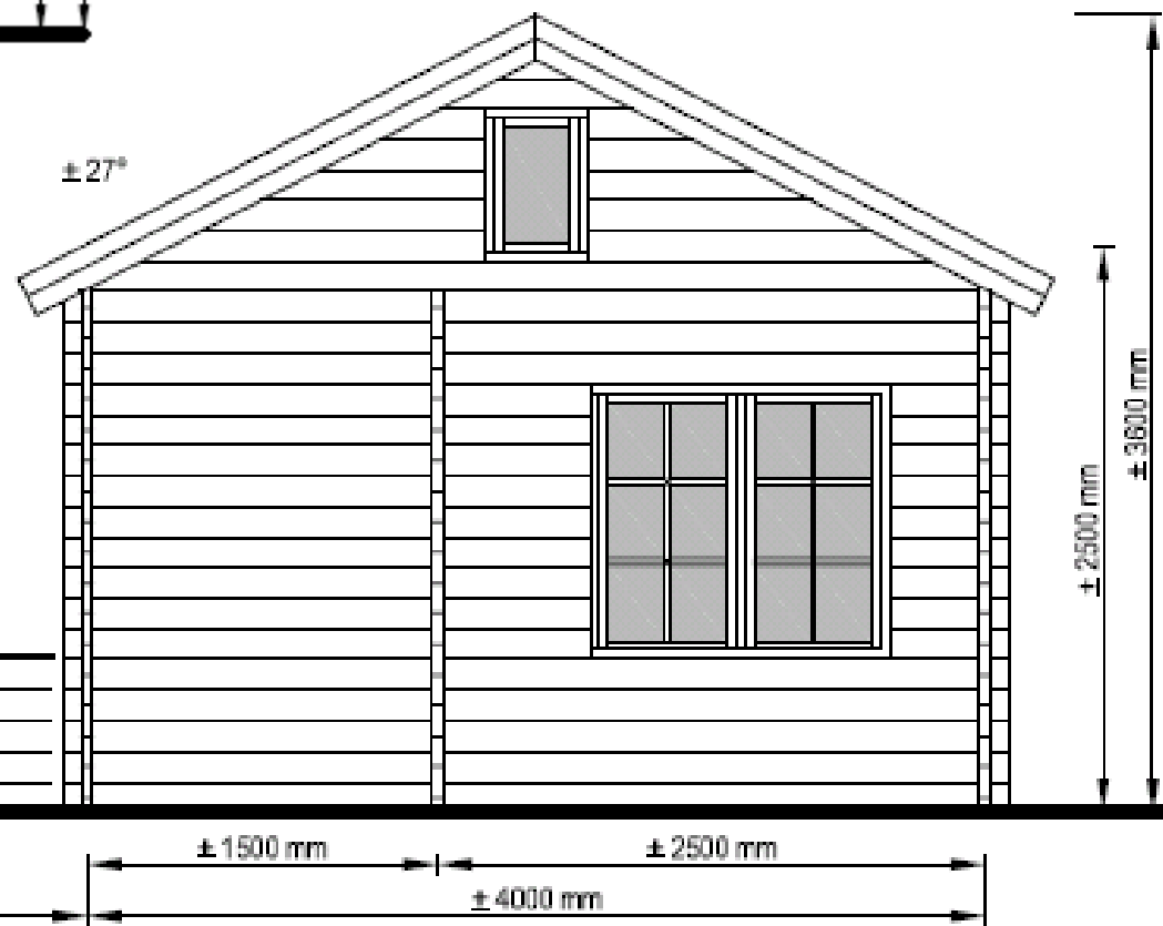
Vooraanzicht
